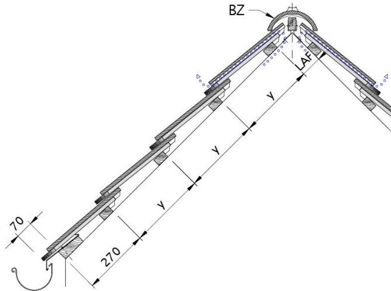
Zeichnung KLASSIK Dachquerschnitt bei Kronendeckung DQK-2
