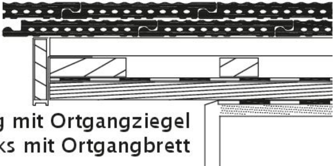
Zeichnung PROFIL Ortgangziegel links mit Ortgangbrett OBL
